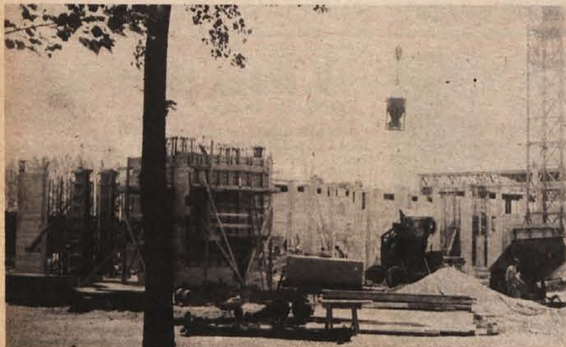
Gradnja objektov za pripravo papirne mase iz odpadnega papirja, ki bo osnovna surovina za nov papirni stroj.
