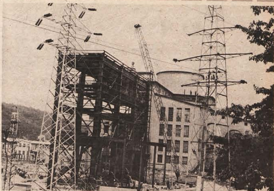
Skupna moč nove plinsko-parne elektrarne v Brestanici bo 94 megawatov, kar je štirikrat več, kot je imela dosedanja, ki so jo poganjali s premogom.
